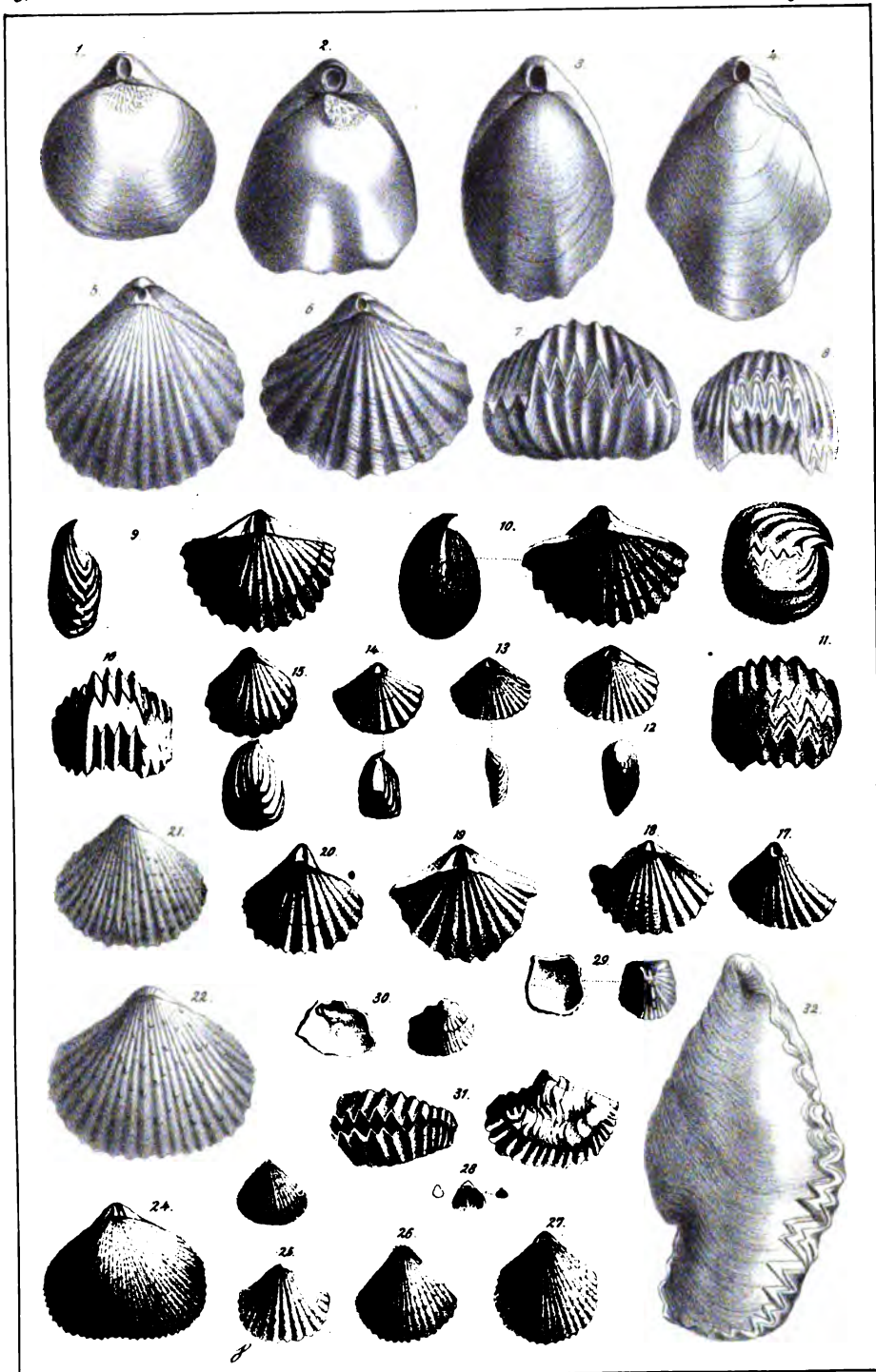
Quenstedt Jura.
